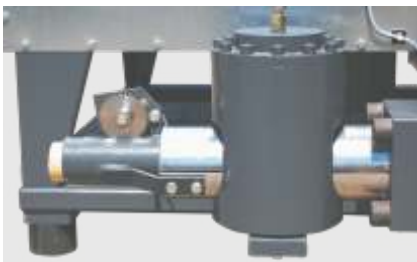
Stranglängenüberwachung zur automatischen Brikettierlängenregulierung
